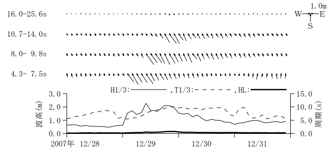
付図-A. 3.36 石巻 周期帯別波浪特性の経時変化(高波期間中)
