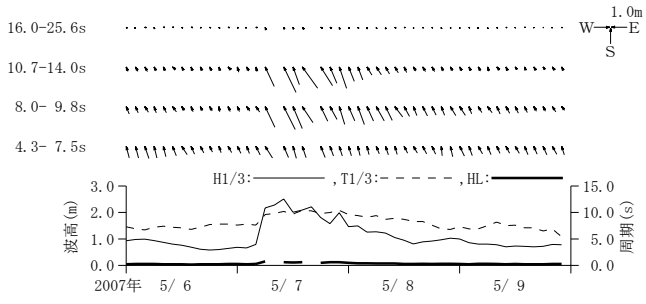
付図-A. 3.36 石巻 周期帯別波浪特性の経時変化(高波期間中)
