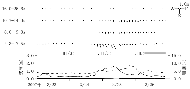
付図-A. 3. 42 第二海堡 周期帯別波浪特性の経時変化(高波期間中)
