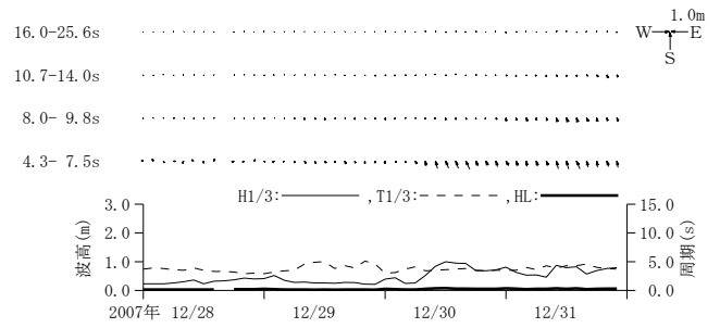
付図-A. 3. 42 第二海堡 周期帯別波浪特性の経時変化(高波期間中)
