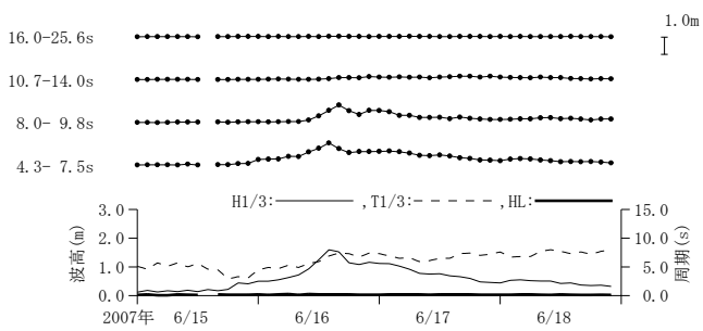
付図-A. 3.34 宮古 周期帯別波浪特性の経時変化(高波期間中)
