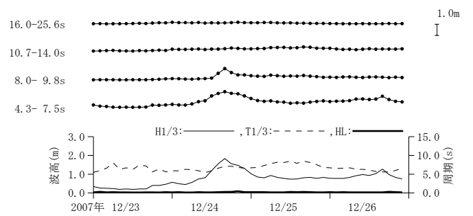
付図-A. 3.34 宮古 周期帯別波浪特性の経時変化(高波期間中)
