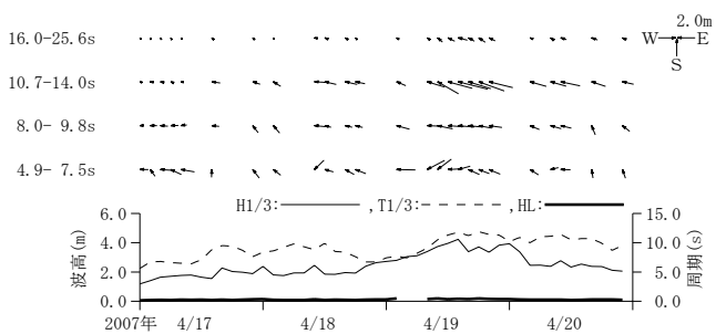
付図-A. 3. 44 波浮 周期帯別波浪特性の経時変化(高波期間中)
