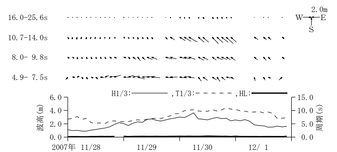
付図-A. 3. 44 波浮 周期帯別波浪特性の経時変化(高波期間中)
