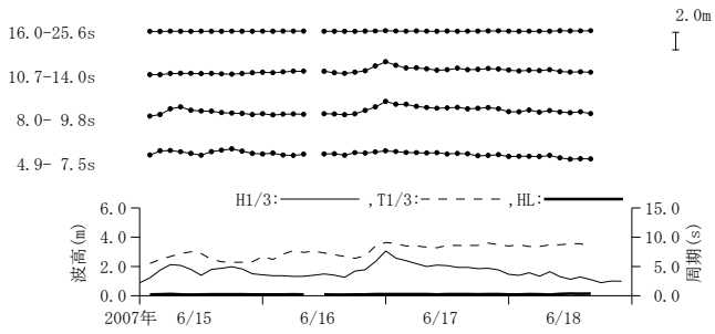
付図-A. 3. 40 常陸那珂 周期帯別波浪特性の経時変化(高波期間中)
