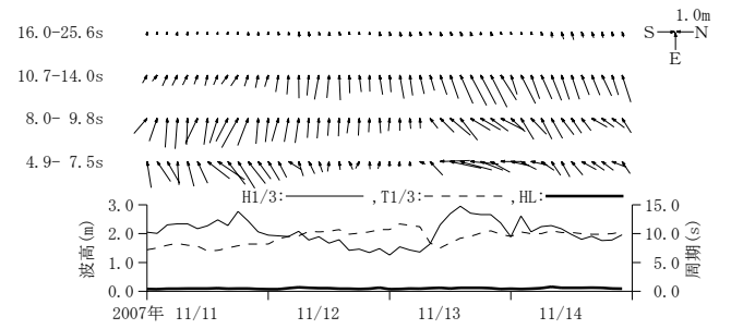
付図-A. 3. 40 常陸那珂 周期帯別波浪特性の経時変化(高波期間中)
