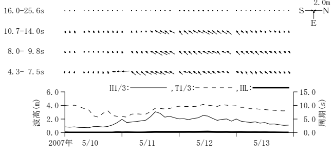
付図-A. 3. 41 鹿島 周期帯別波浪特性の経時変化(高波期間中)
