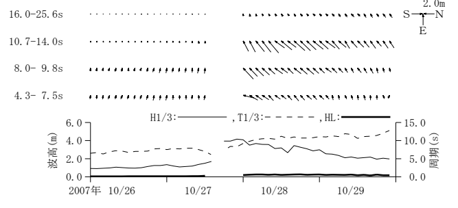
付図-A. 3. 41 鹿島 周期帯別波浪特性の経時変化(高波期間中)
