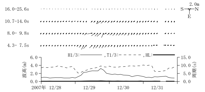
付図-A. 3. 39 小名浜 周期帯別波浪特性の経時変化(高波期間中)
