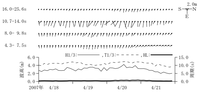
付図-A. 3. 39 小名浜 周期帯別波浪特性の経時変化(高波期間中)
