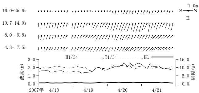
付図-A. 3.37 仙台新港 周期帯別波浪特性の経時変化(高波期間中)
