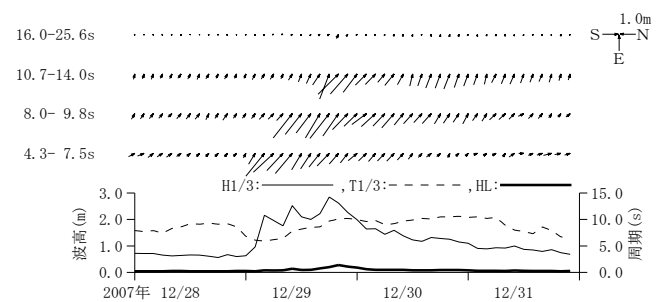
付図-A. 3.37 仙台新港 周期帯別波浪特性の経時変化(高波期間中)
