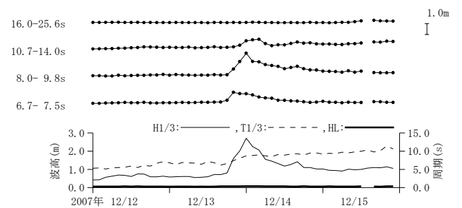
付図-A. 3.35 釜石 周期帯別波浪特性の経時変化(高波期間中)
