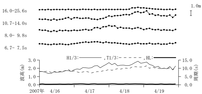
付図-A. 3.35 釜石 周期帯別波浪特性の経時変化(高波期間中)
