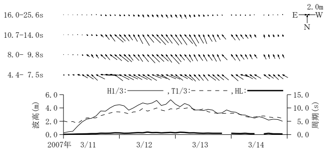
付図-A.3.9 直江津 周期帯別波浪特性の経時変化(高波期間中)
