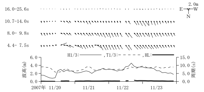
付図-A.3.9 直江津 周期帯別波浪特性の経時変化(高波期間中)
