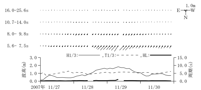
付図-A. 3.11 伏木富山 周期帯別波浪特性の経時変化(高波期間中)
