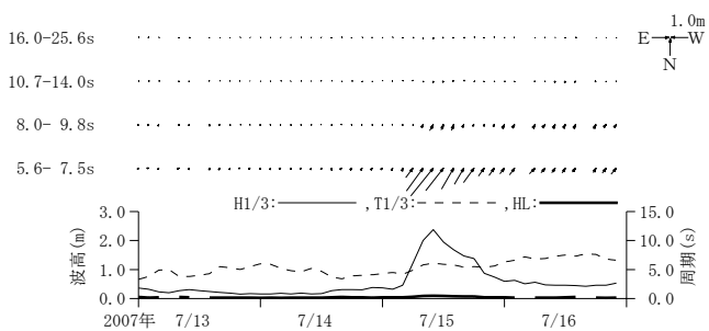
付図-A. 3.11 伏木富山 周期帯別波浪特性の経時変化(高波期間中)
