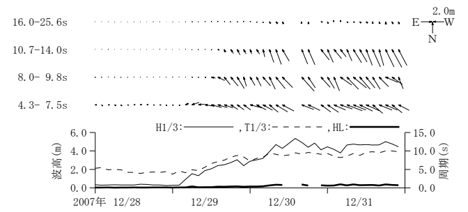
付図-A. 3. 13 金沢 周期帯別波浪特性の経時変化(高波期間中)
