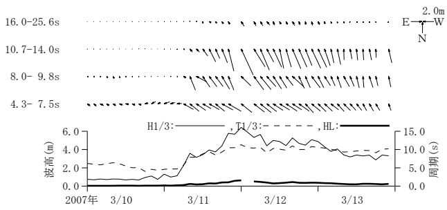
付図-A. 3. 13 金沢 周期帯別波浪特性の経時変化(高波期間中)
