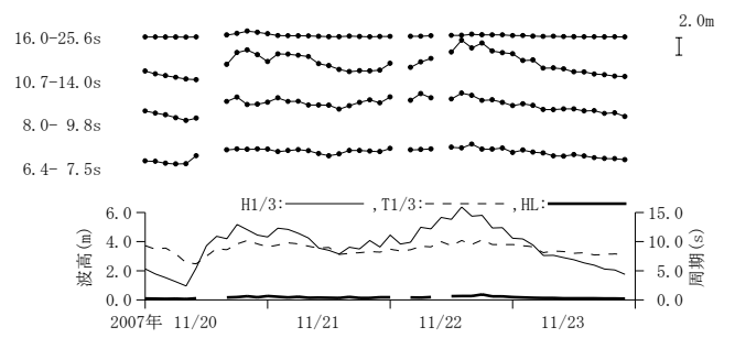
付図-A.3.7 酒田 周期帯別波浪特性の経時変化(高波期間中)
