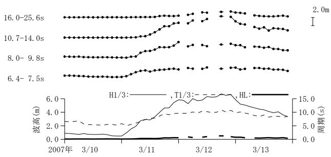
付図-A.3.7 酒田 周期帯別波浪特性の経時変化(高波期間中)
