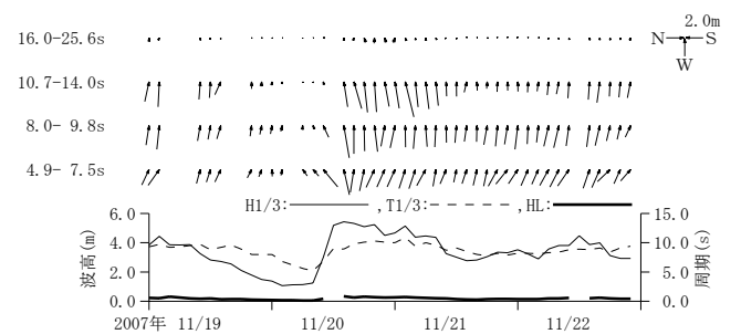
付図-A.3.6 秋田 周期帯別波浪特性の経時変化(高波期間中)
