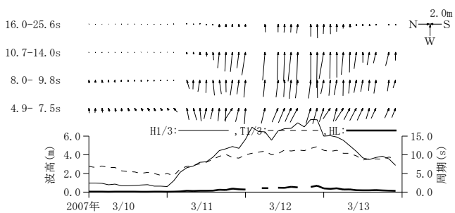
付図-A.3.6 秋田 周期帯別波浪特性の経時変化(高波期間中)
