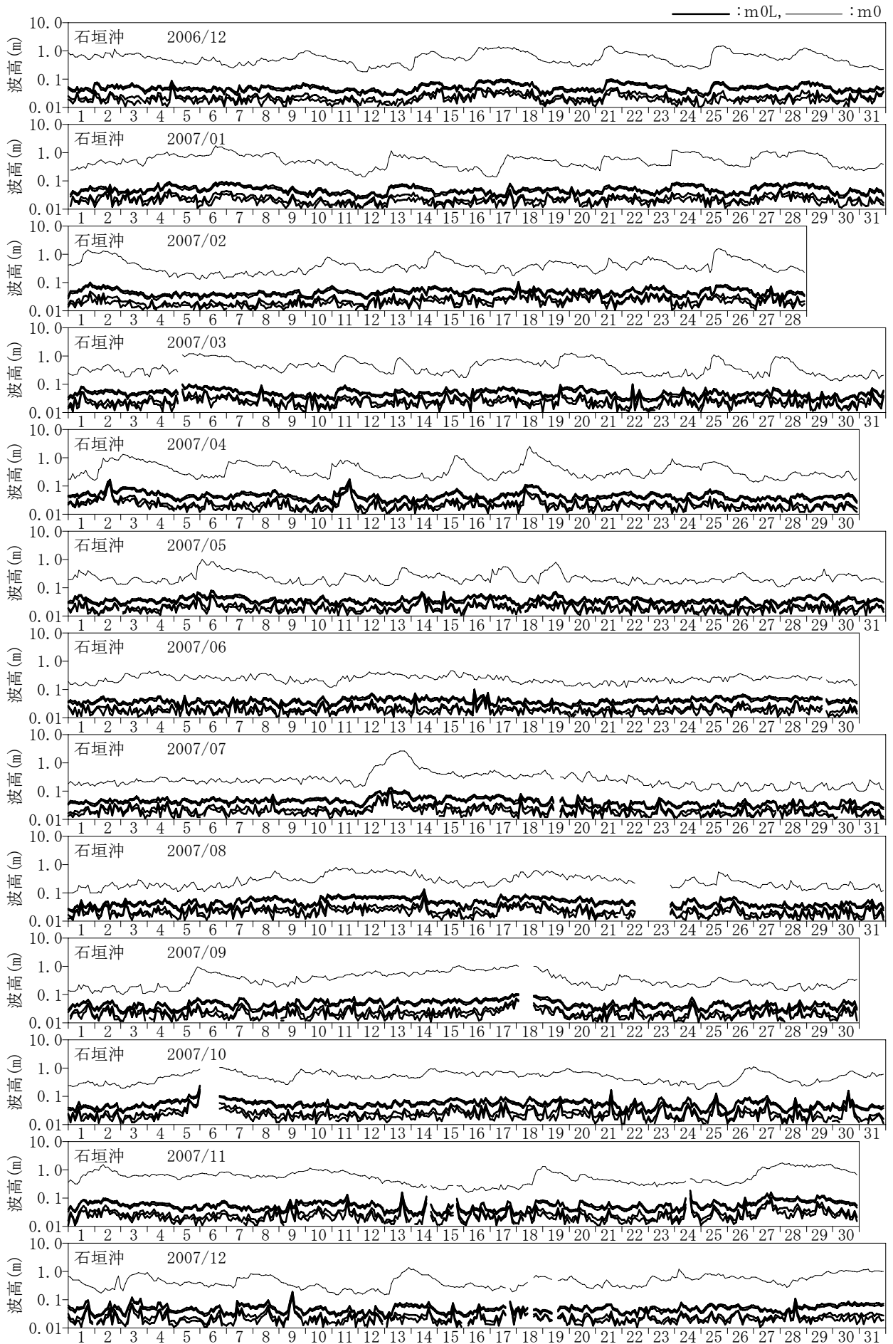
付図-C.1.61 長周期波高の経時変化図 (石垣沖)
