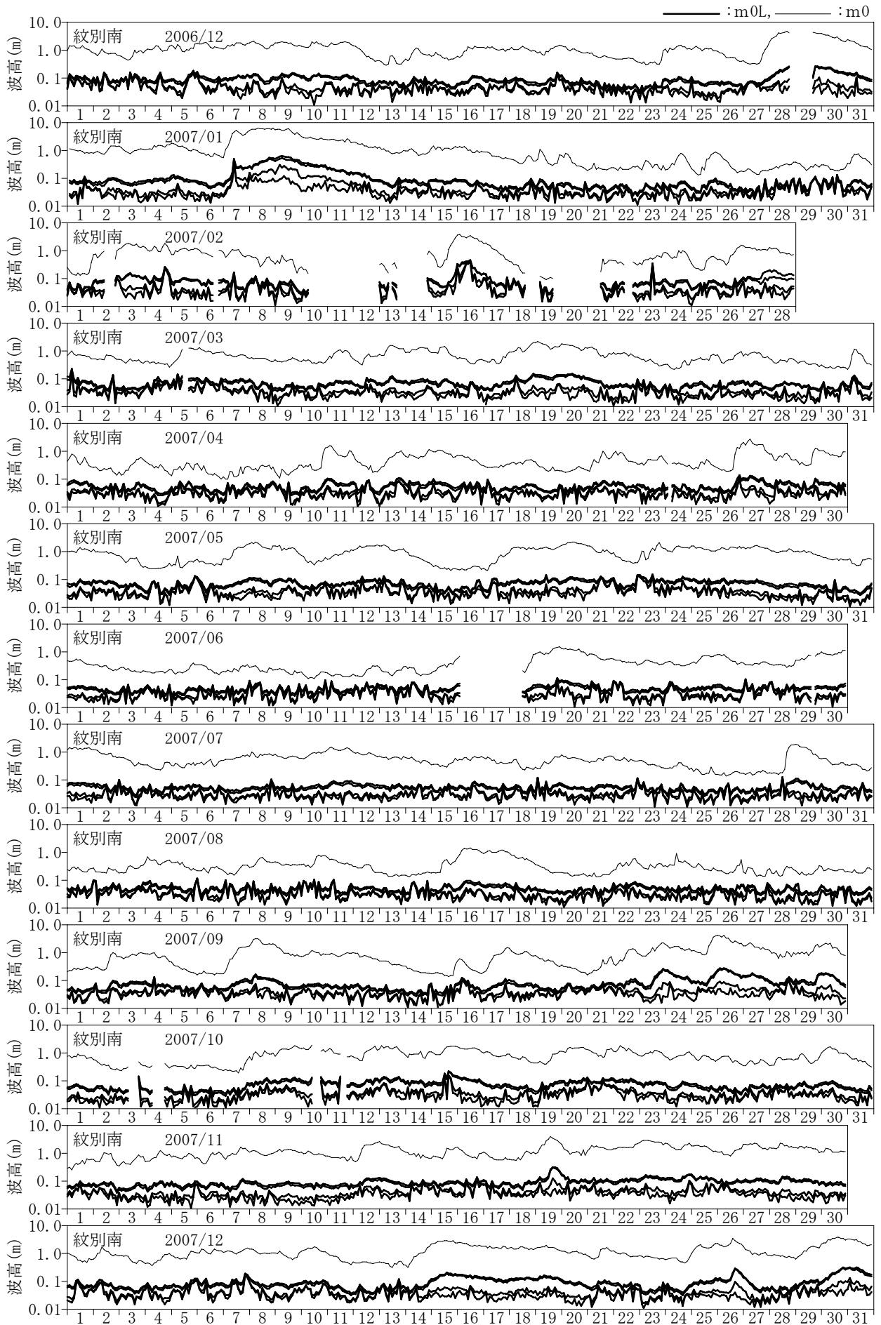
付図-C.1.27 長周期波高の経時変化図 (紋別(南))
