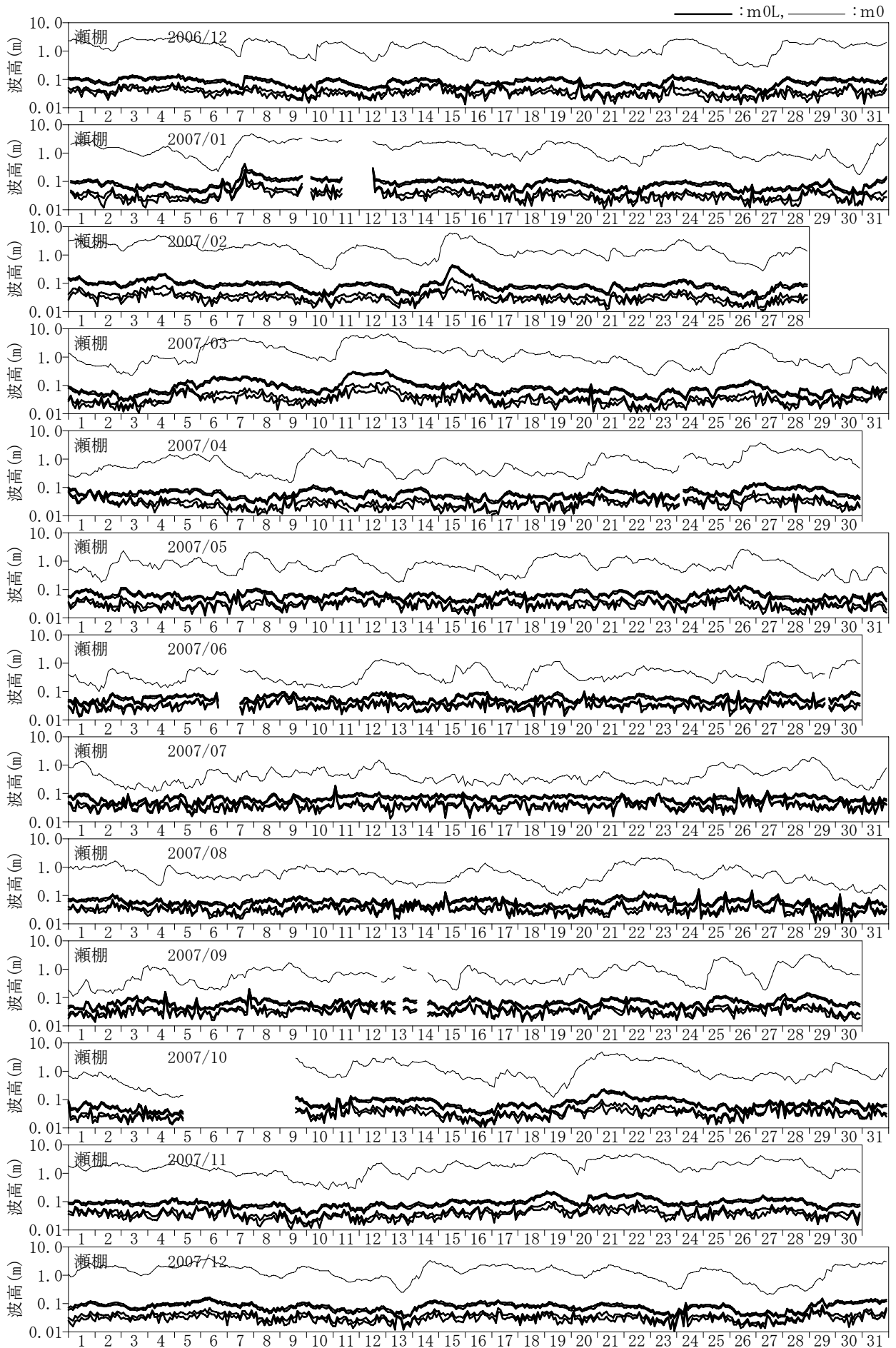
付図-C.1.3 長周期波高の経時変化図 (瀬棚)
