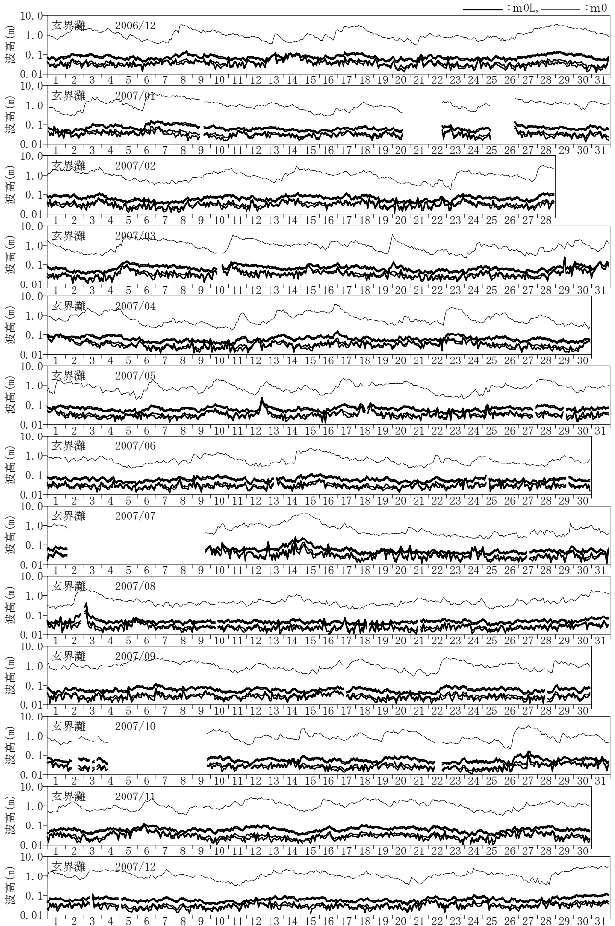
付図-C.1.22 長周期波高の経時変化図 (玄界灘)
