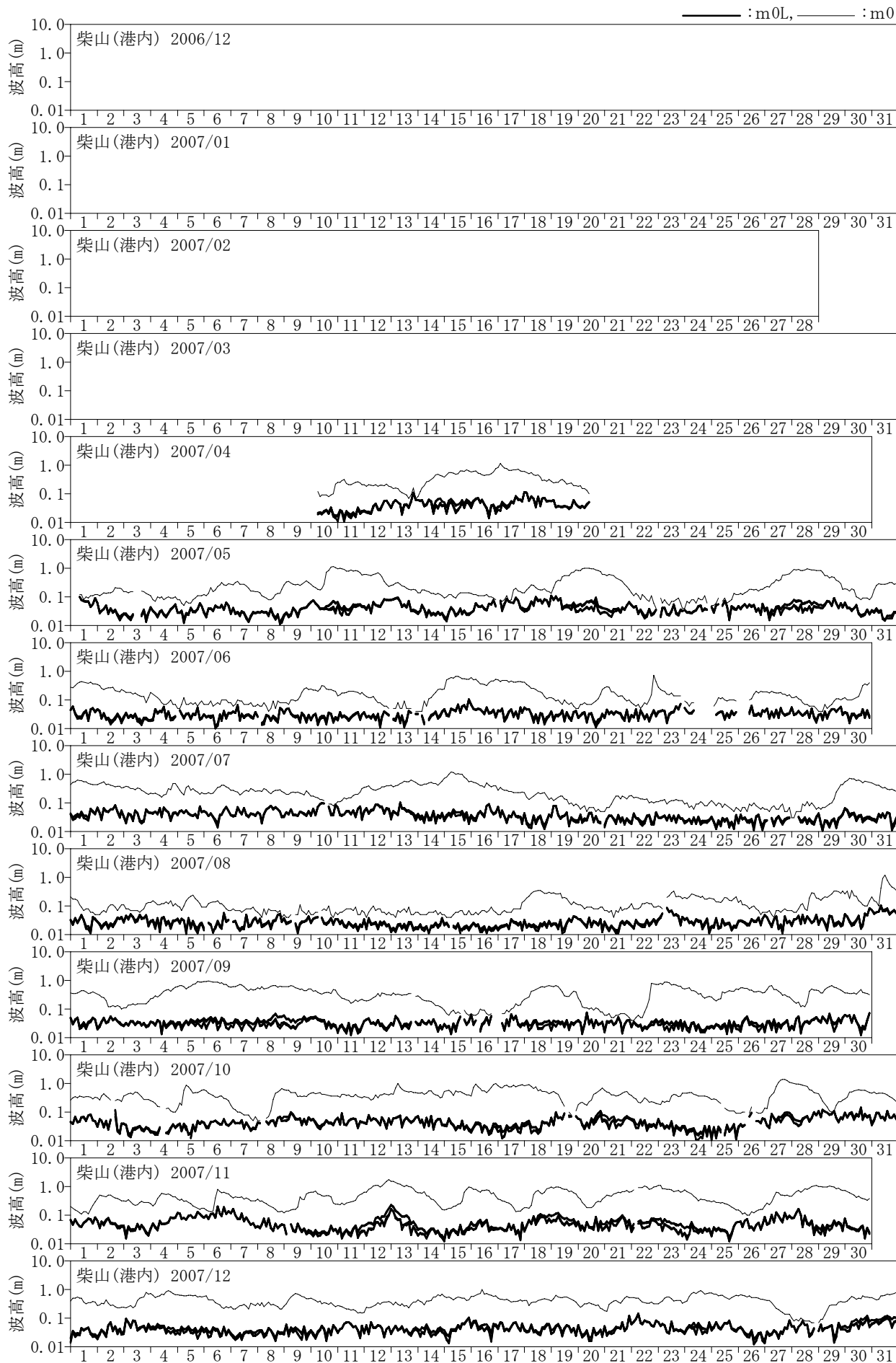
付図-C.1.17 長周期波高の経時変化図 (柴山(港内))
