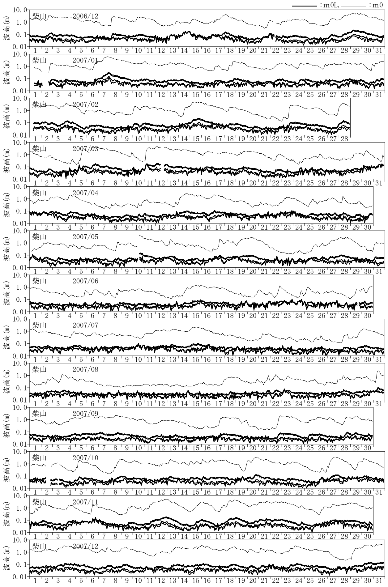
付図-C.1.16 長周期波高の経時変化図 (柴山)
