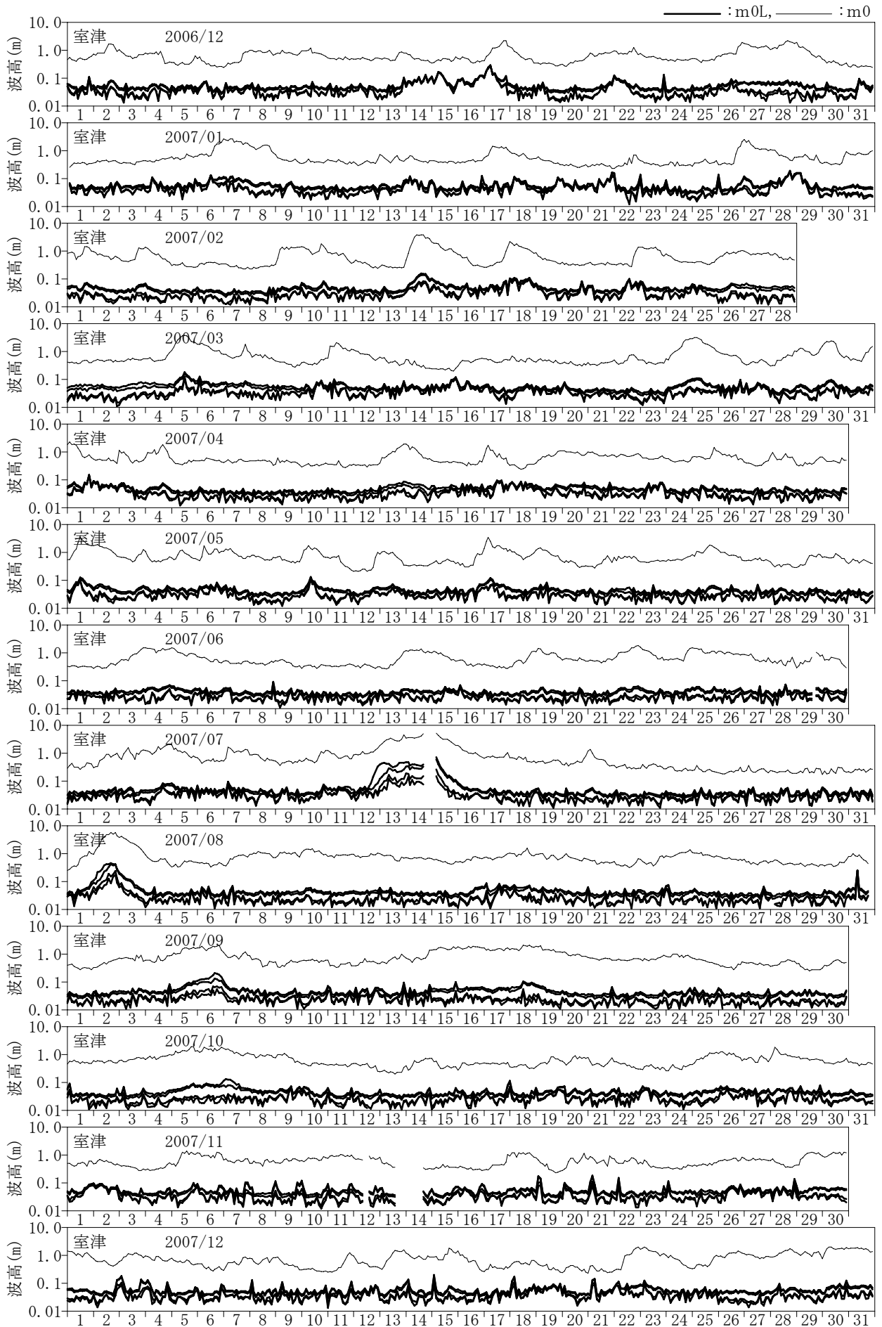
付図-C.1.52 長周期波高の経時変化図 (室津)
