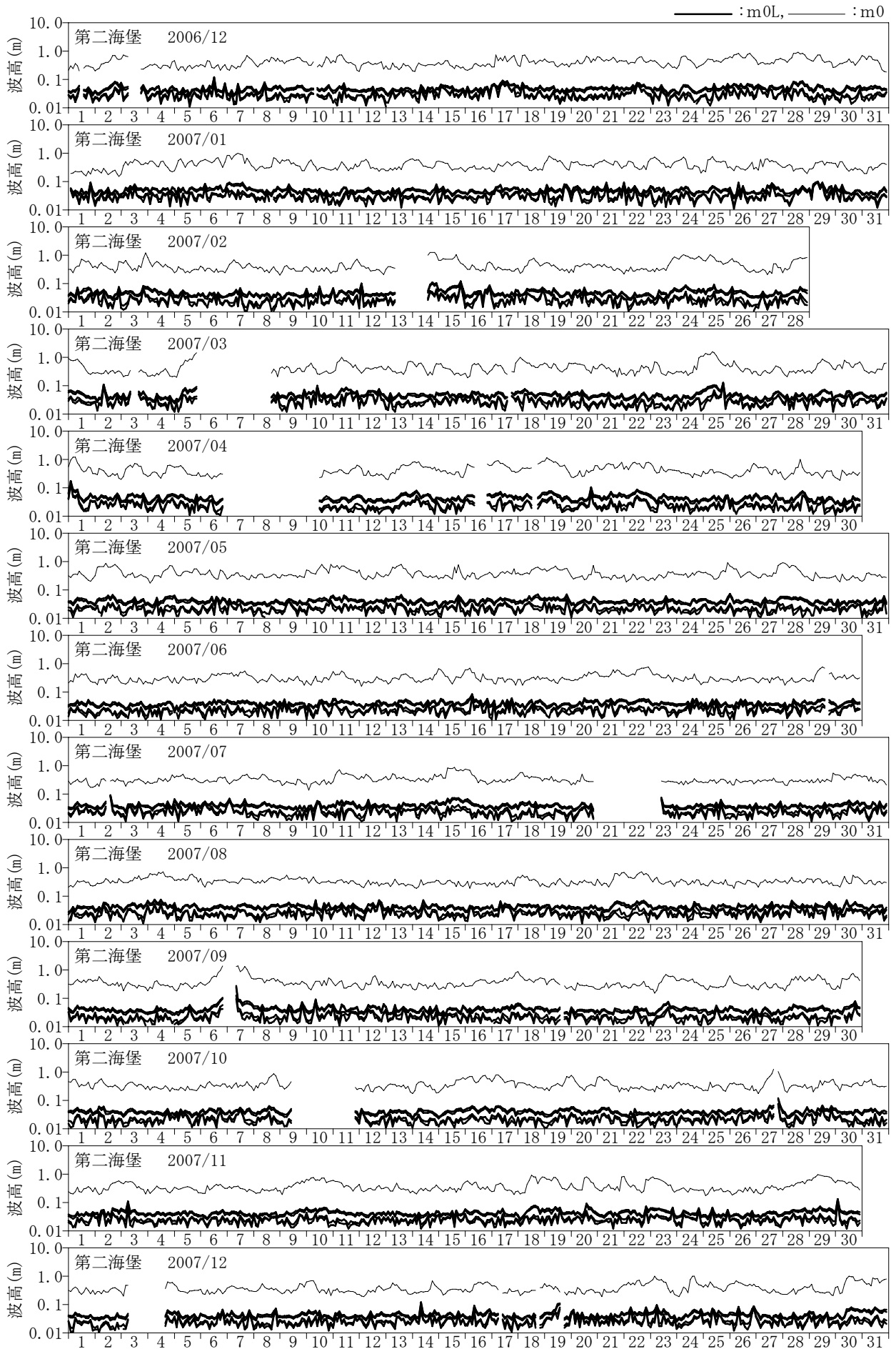
付図-C.1.42 長周期波高の経時変化図 (第二海堡)
