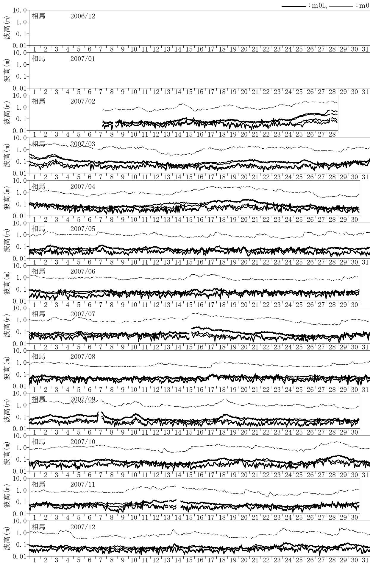
付図-C.1.38 長周期波高の経時変化図 (相馬)
