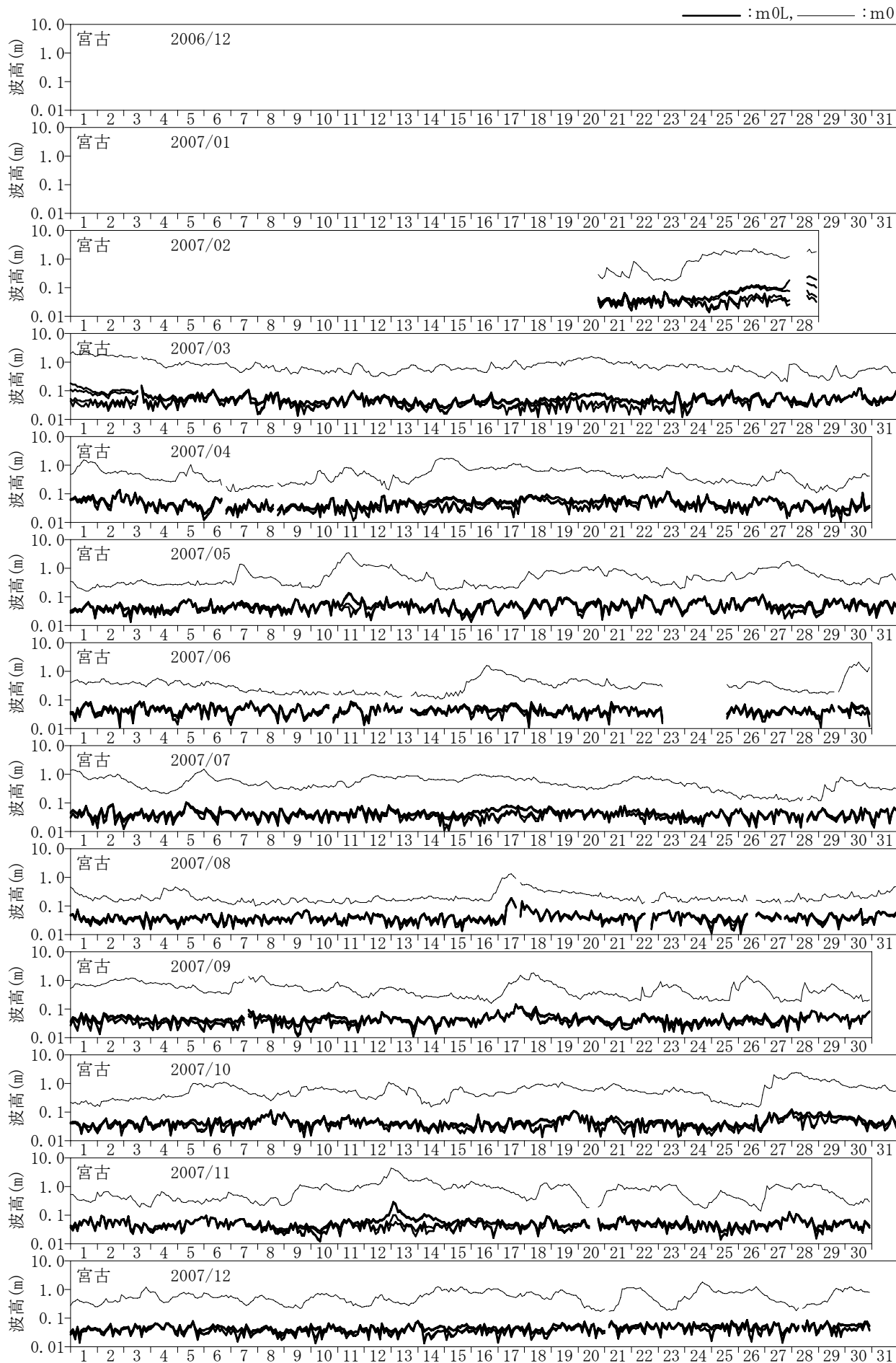
付図-C.1.34 長周期波高の経時変化図 (宮古)
