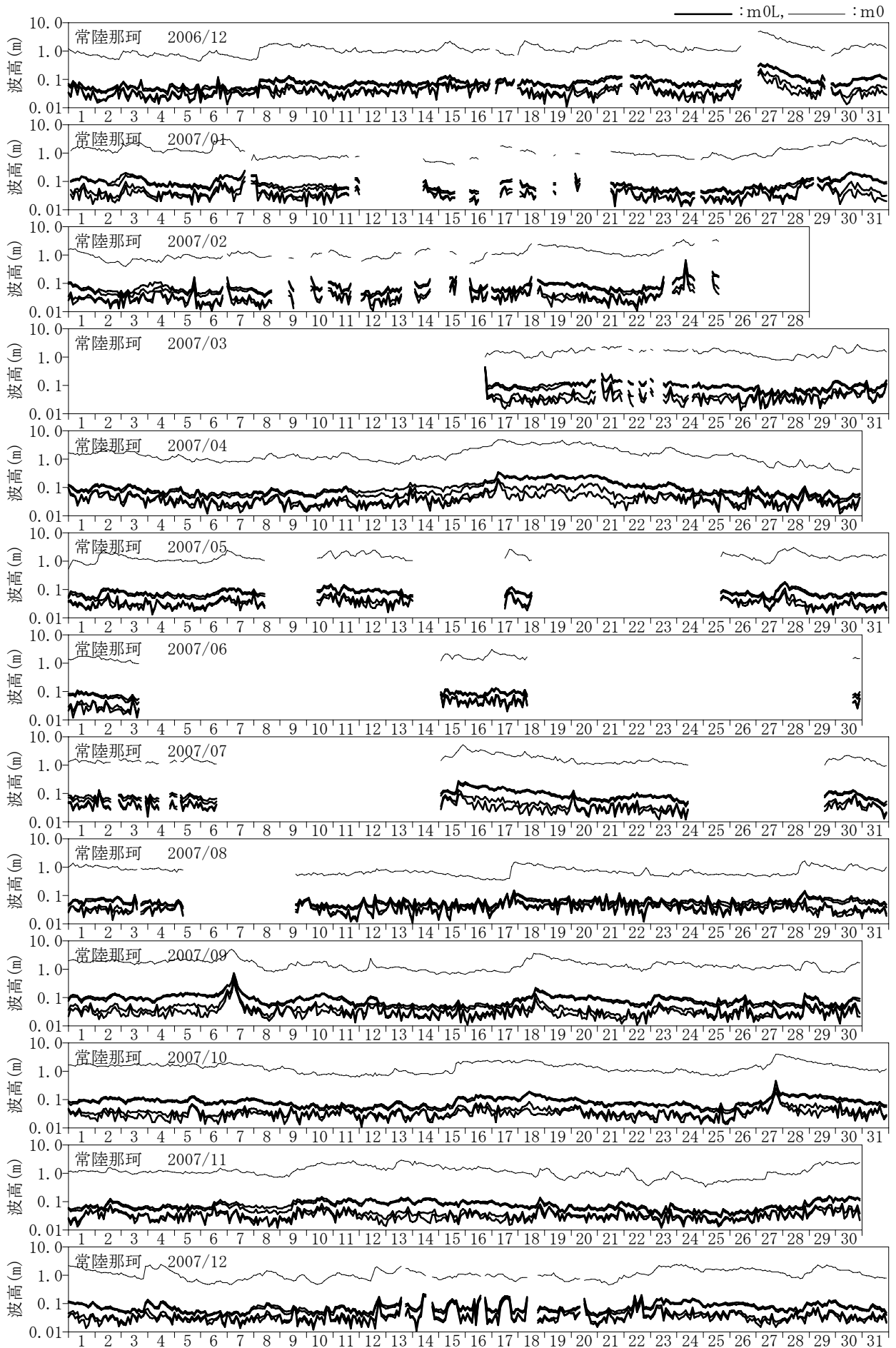
付図-C.1.40 長周期波高の経時変化図 (常陸那珂)
