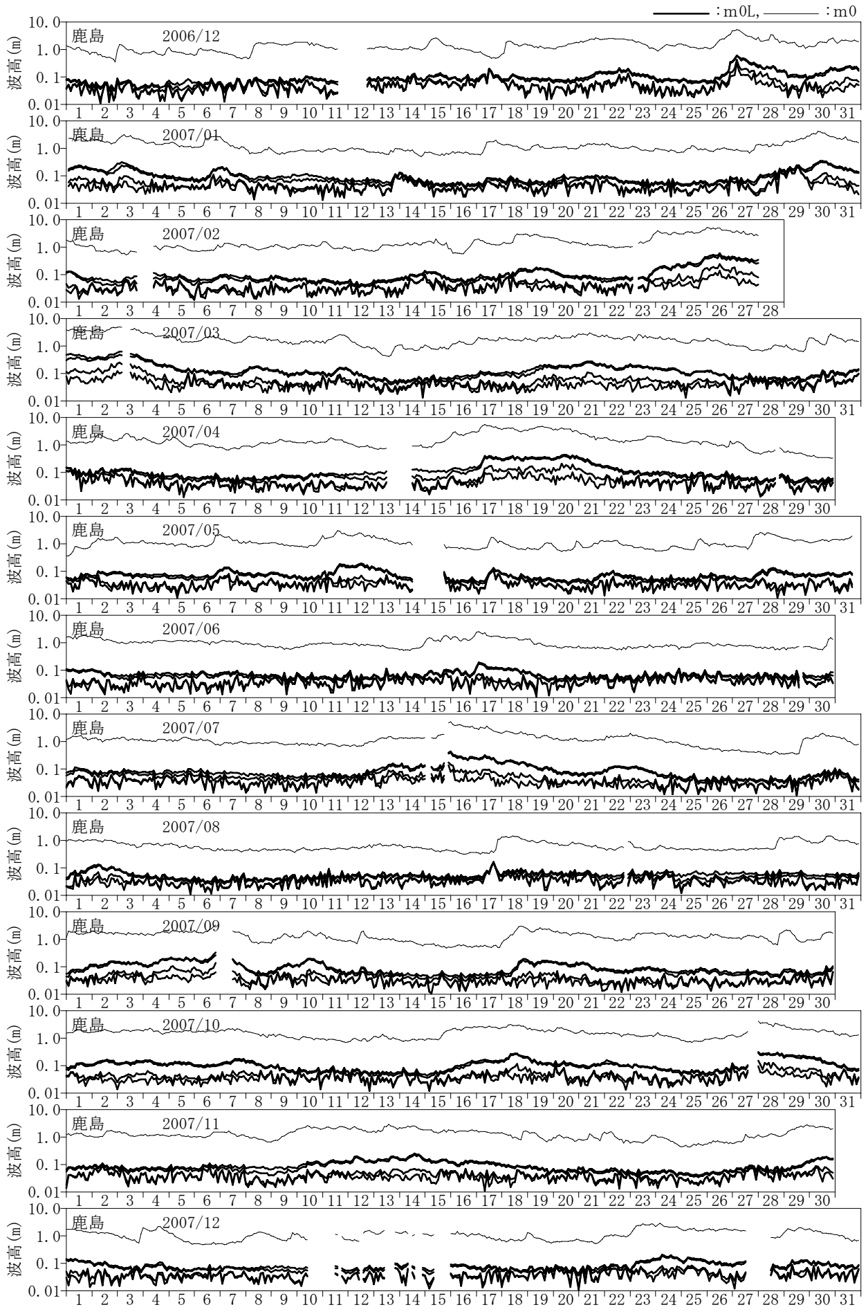
付図-C.1.41 長周期波高の経時変化図 (鹿島)
