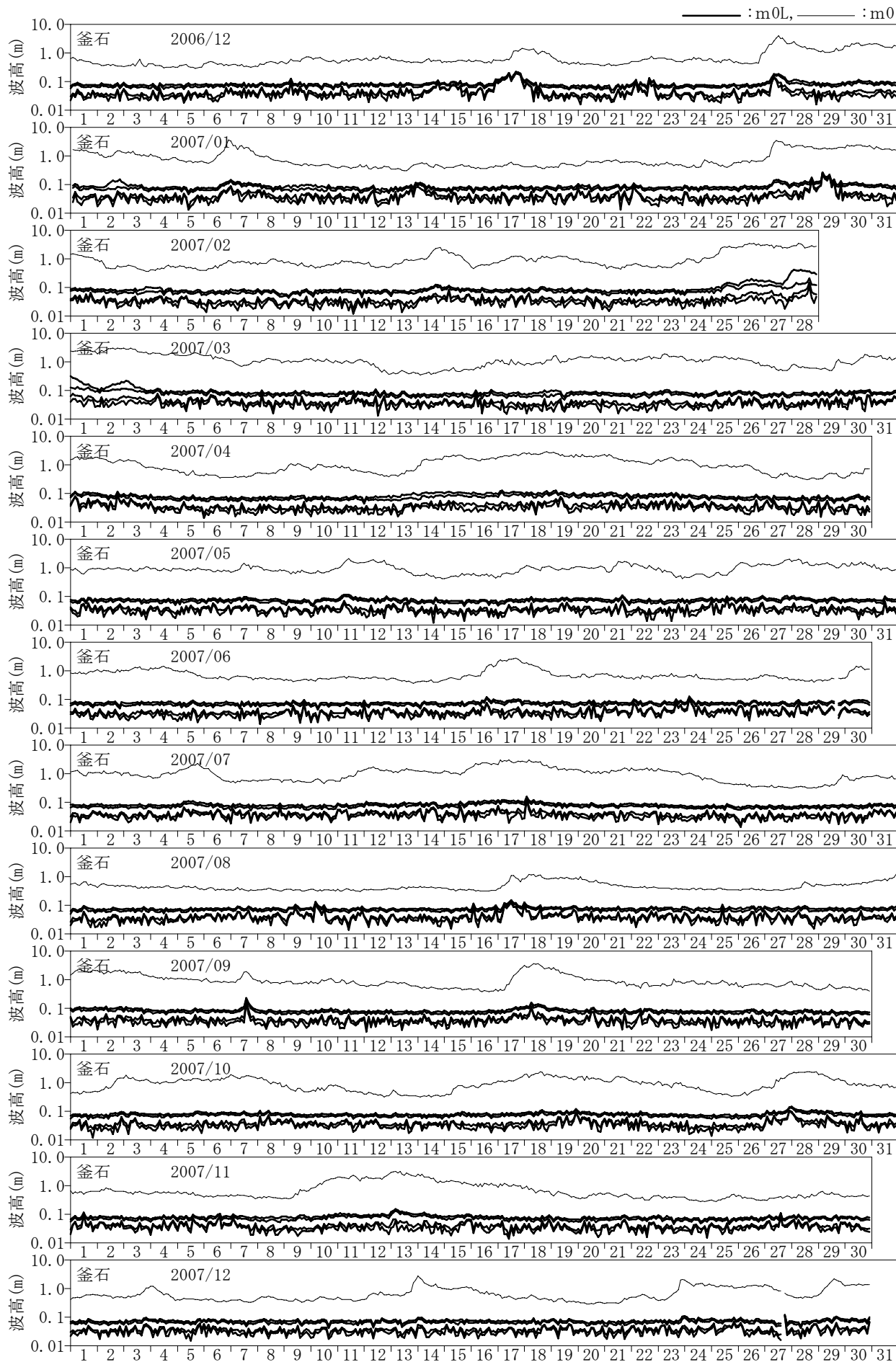
付図-C.1.35 長周期波高の経時変化図 (釜石)
