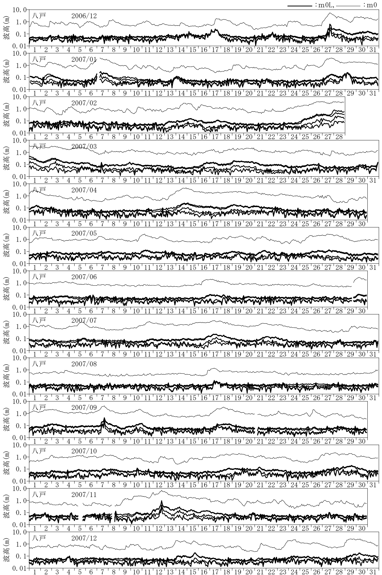
付図-C.1.32 長周期波高の経時変化図 (八戸)
