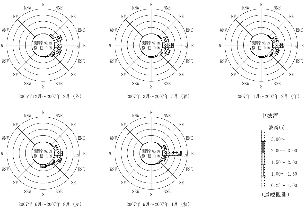
付図-B.2.59 中城湾 波高・波向別出現頻度図 (連続観測)
