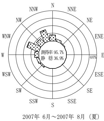
付図-B.2.2 石狩新港 波高・波向別出現頻度図（連続観測）
