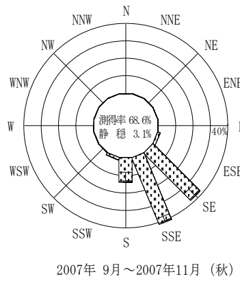
付図-B.2.53 高知 波高・波向別出現頻度図（連続観測）
