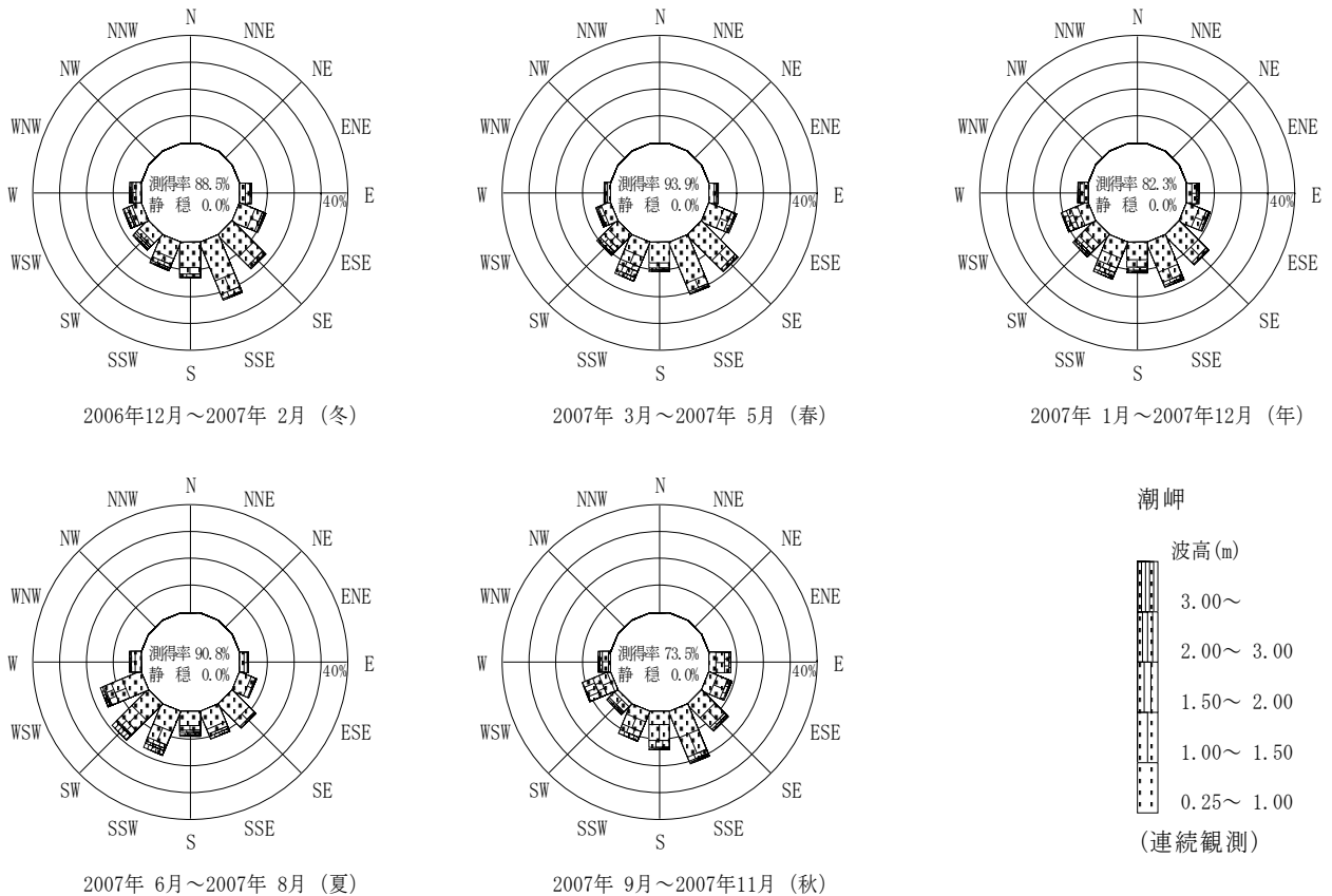
付図-B.2.49 潮岬 波高・波向別出現頻度図（連続観測）
