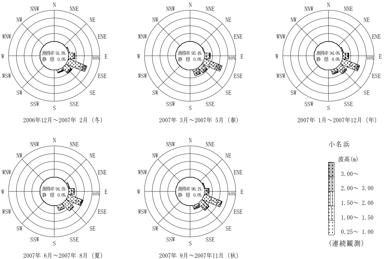
付図-B.2.39 小名浜 波高・波向別出現頻度図(連続観測)
