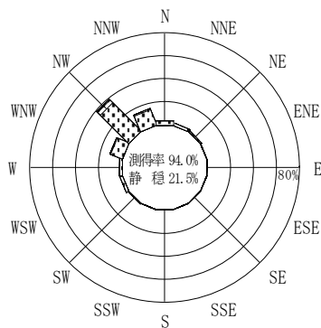
付図-A.2.61 石垣沖 波高・波向別出現頻度図
