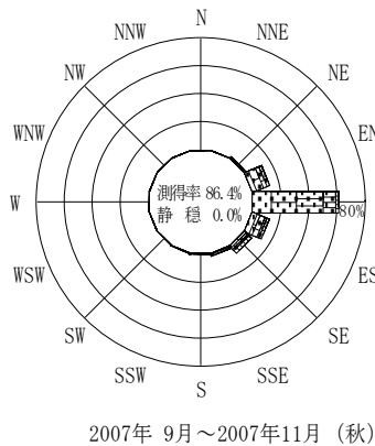
付図-A.2.59 中城湾 波高・波向別出現頻度図
