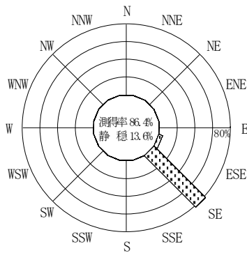
付図-A.2.51 小松島 波高・波向別出現頻度図
