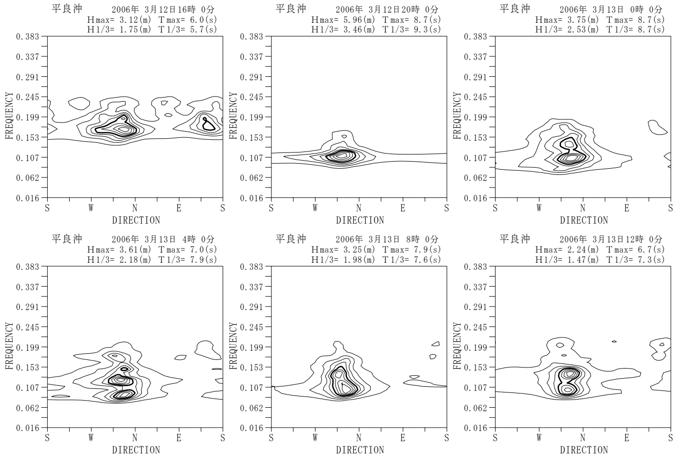
付図-A. 5. 60 平良沖 代表的な高波期間中の方向スペクトル
