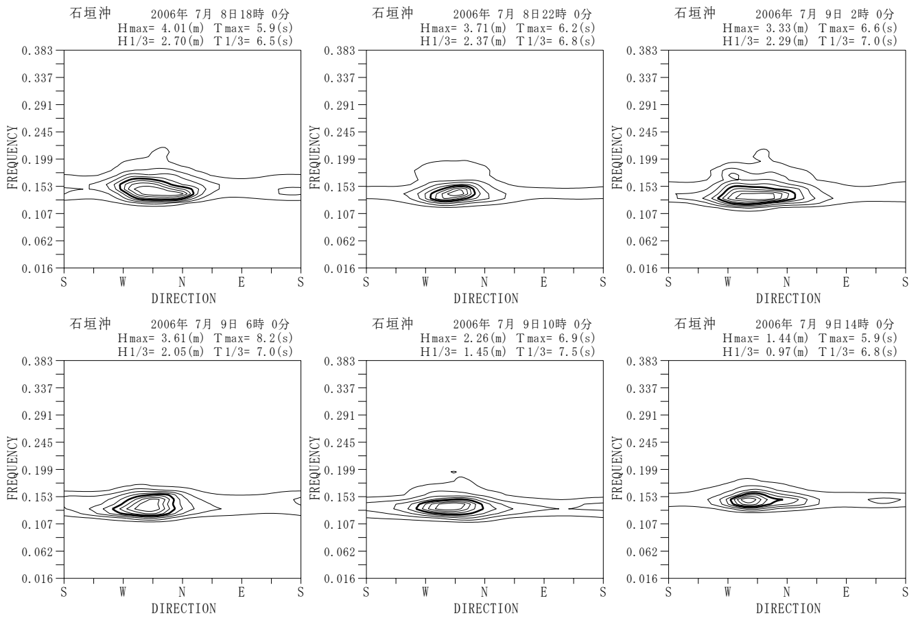
付図-A. 5. 62 石垣沖 代表的な高波期間中の方向スペクトル
