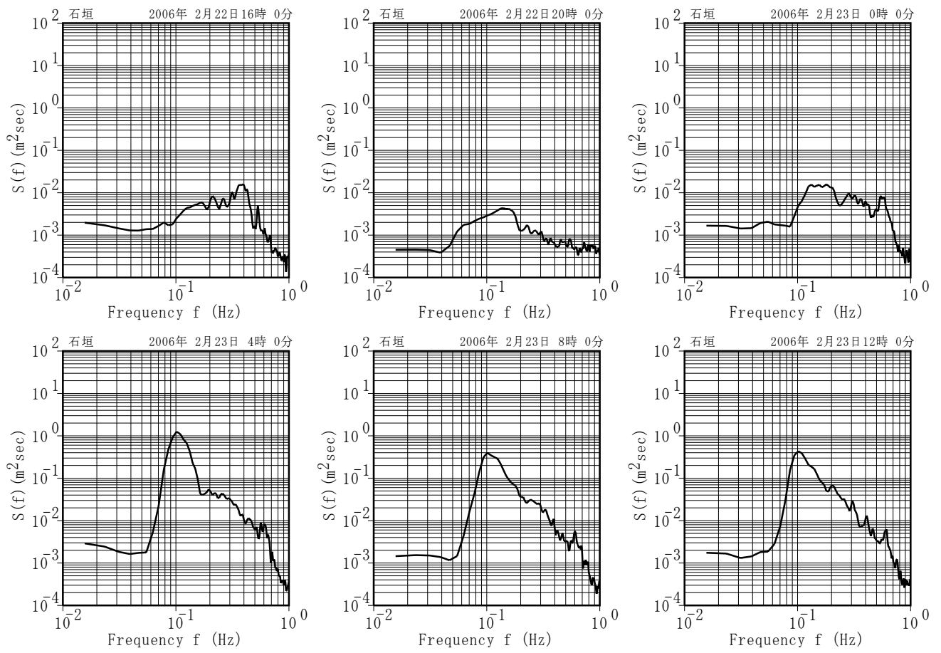
付図-A.5.61 石垣 代表的な高波期間中のスペクトル
