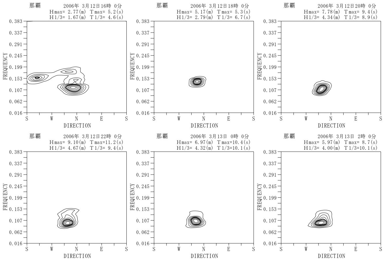
付図-A. 5. 26 那覇 代表的な高波期間中の方向スペクトル
