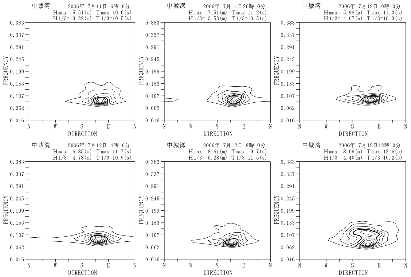
付図-A. 5.59 中城湾 代表的な高波期間中の方向スペクトル
