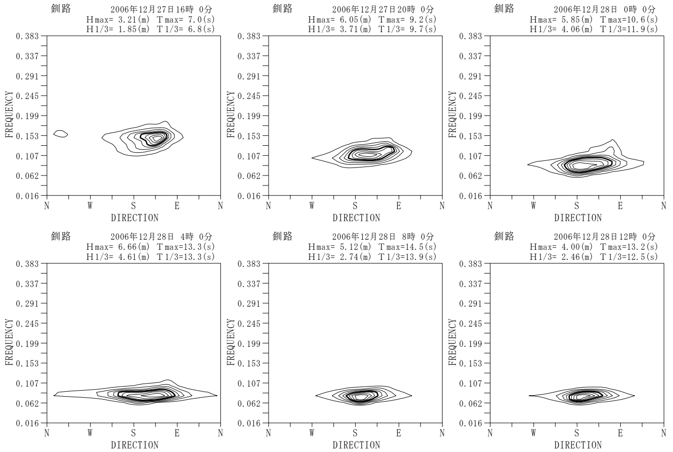
付図-A. 5. 28 釧路 代表的な高波期間中の方向スペクトル
