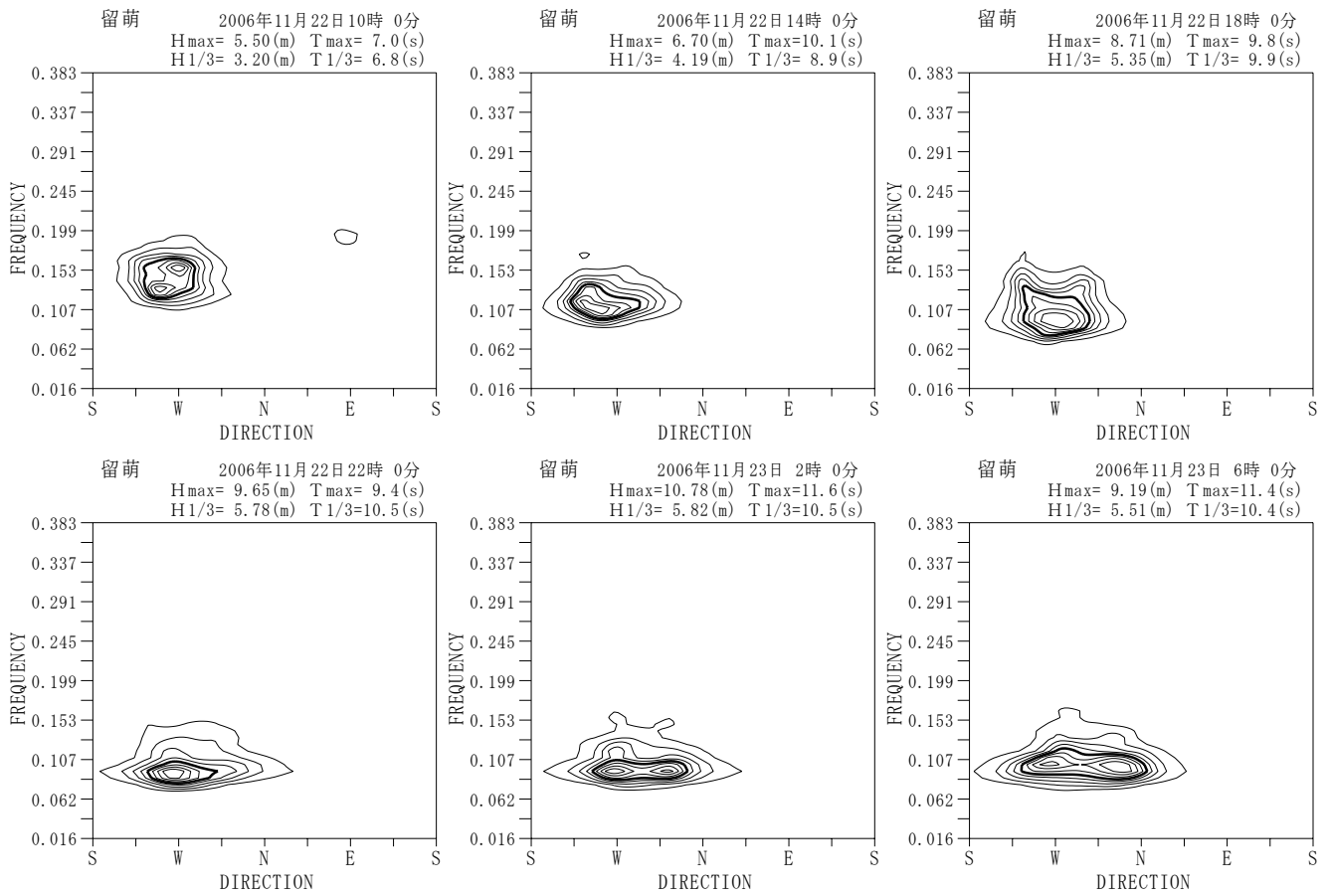
付図-A.5.1 留萌 代表的な高波期間中の方向スペクトル
