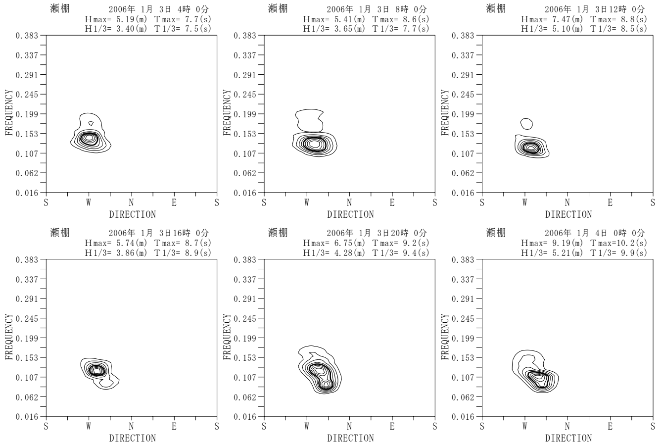
付図-A.5.3 瀬棚 代表的な高波期間中の方向スペクトル
