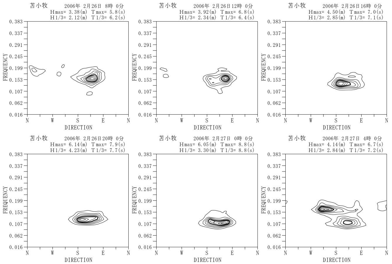
付図-A. 5. 30 苦小牧 代表的な高波期間中の方向スペクトル
