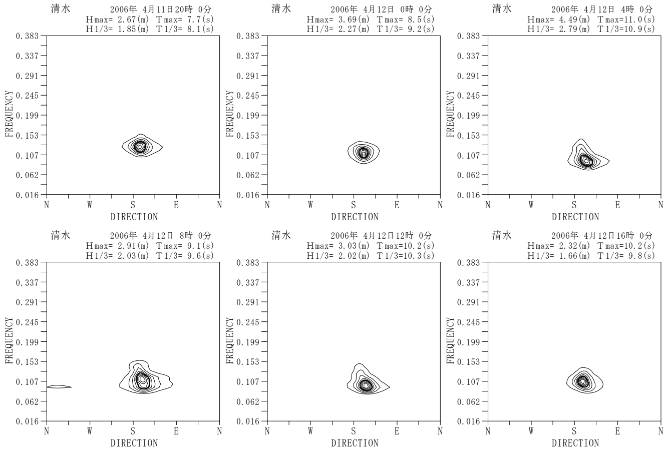
付図-A. 5. 45 清水 代表的な高波期間中の方向スペクトル
