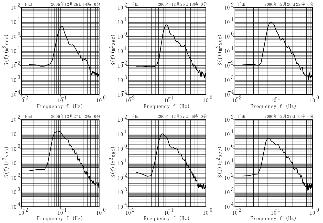
付図-A.5.44 下田 代表的な高波期間中のスペクトル
