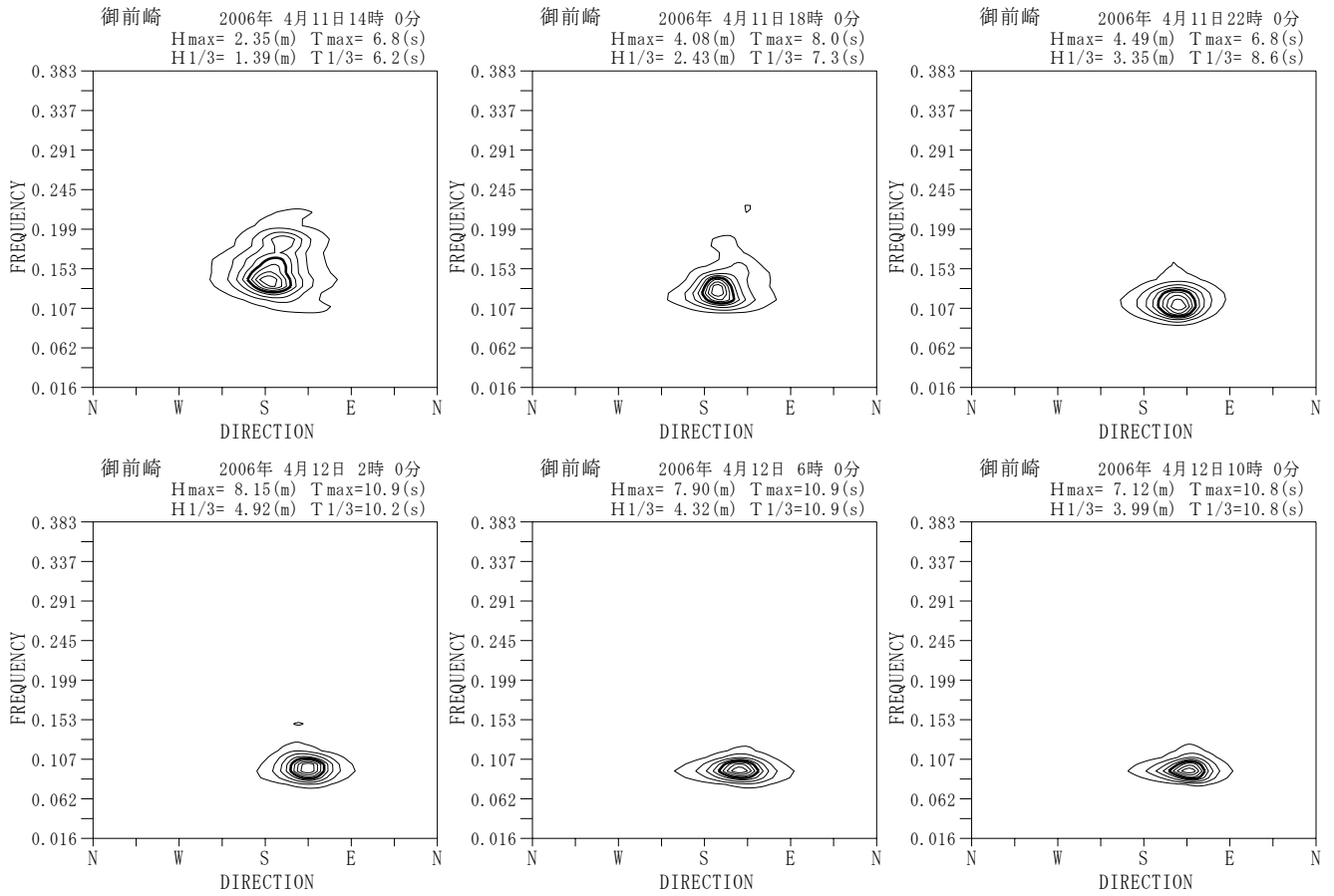
付図-A. 5. 46 御前崎 代表的な高波期間中の方向スペクトル
