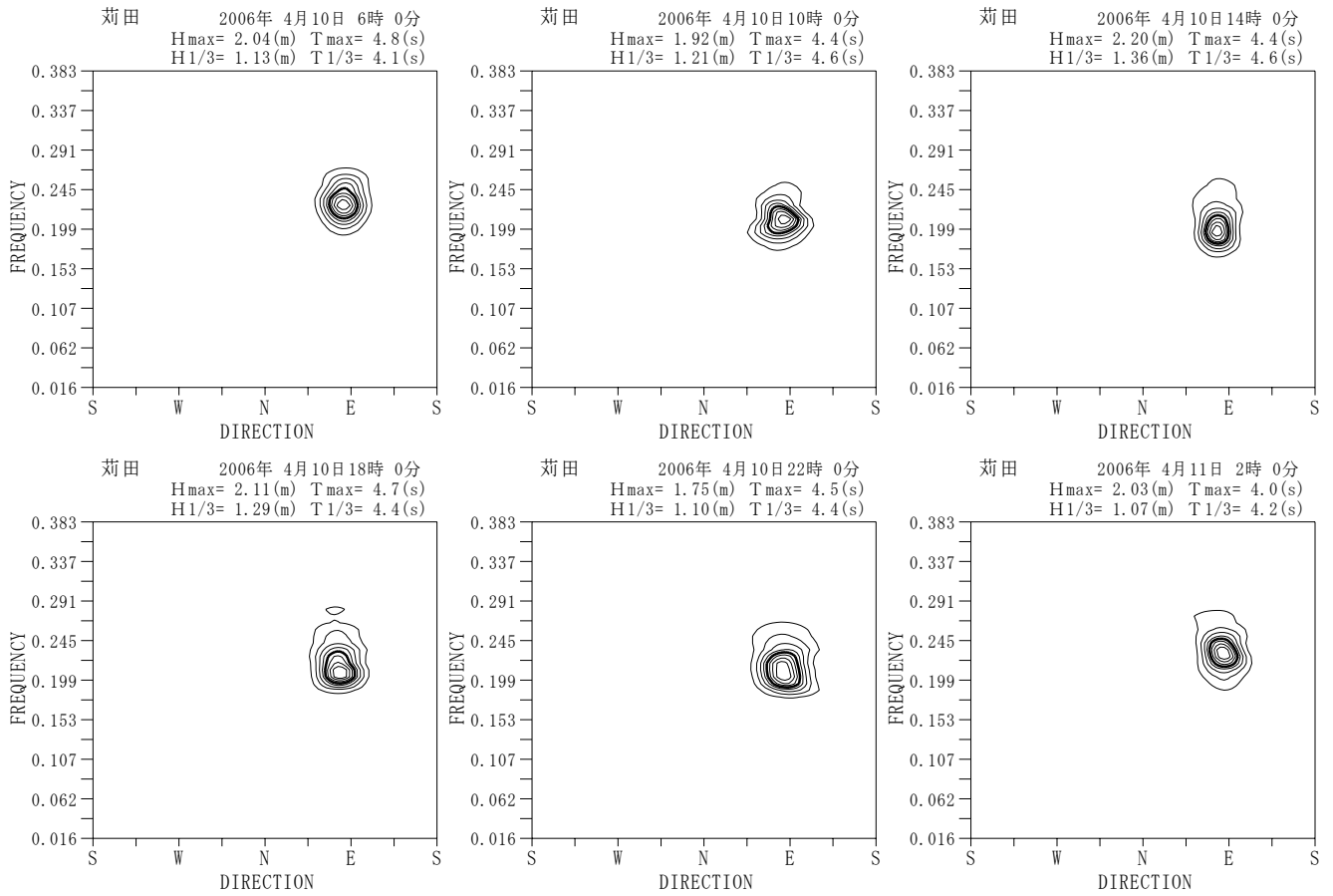
付図-A. 5.55 荻田 代表的な高波期間中の方向スペクトル
