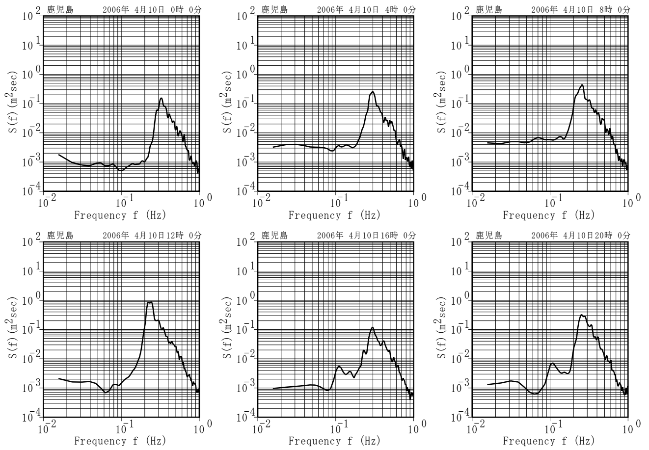
付図-A. 5. 58 鹿児島 代表的な高波期間中のスペクトル
